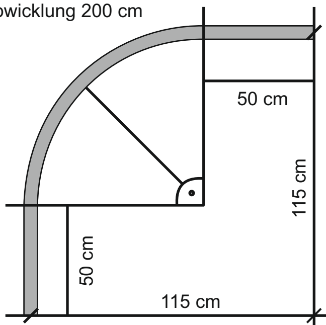
Norm-Kreisbogen 90° Profil 100
