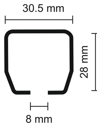
Querschnitt Profil Modell 100
