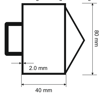
Querschnitt des Querträgers ab 6 m Seitenlänge inkl. Verstärkung auf der ganzen Länge
