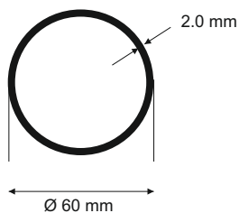
Querschnitt der Firsttraverse für alle Zelt
