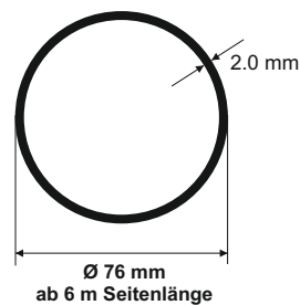
Querschnitt der Fusstütze ab 6 m Seitenlänge
