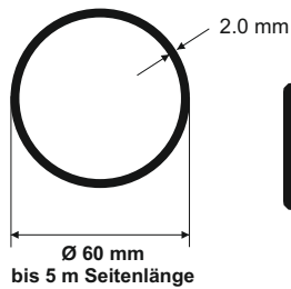
Querschnitt der Fusstütze bis 5 m Seitenlänge
