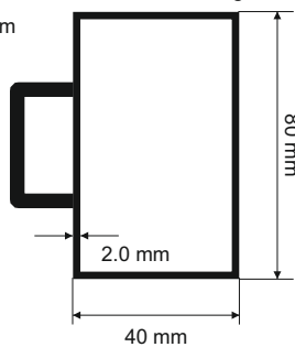
Querschnitt des Querträgers bis 5 m Seitenlänge
